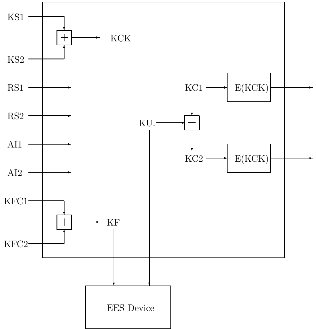
Fig. 3. EES Key Generation
